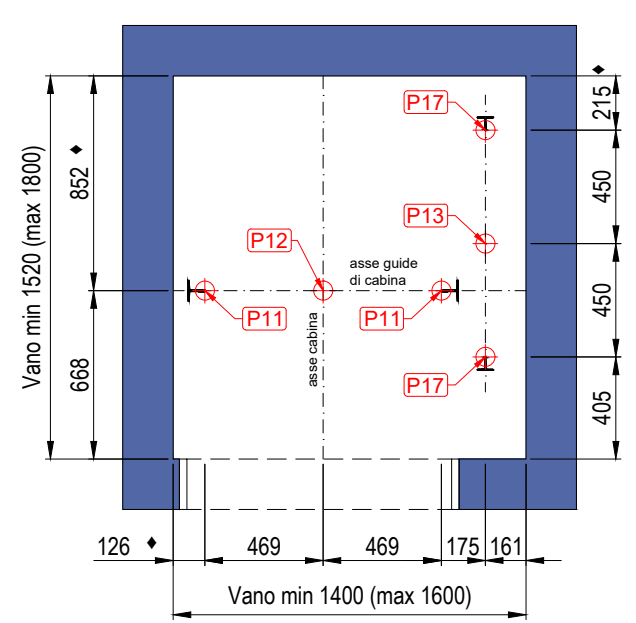
CARICHI ACCIDENTALI IN FOSSA (daN)
